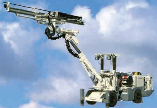
1ブームホイールドリルジャンボ JTH1AM-210
