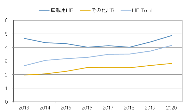
図 2-2-3 国内生産 LIB の 1 個当たり容量(Ah/個)
