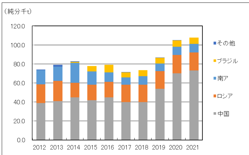
図 2-1 世界のバナジウム鉱石の生産量
