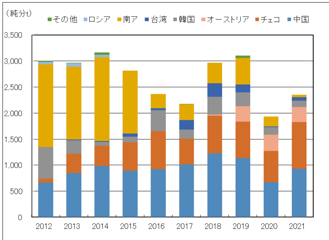
図 3-2-1 FeV の輸入相手国
